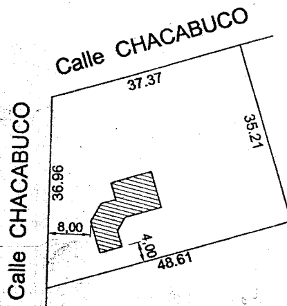
Croquis de Emplazamiento
